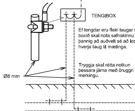
SNÍÐ Í TÖFLUVEGG
