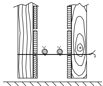
SNÍÐ A - A Í SÖKKULVEGG
